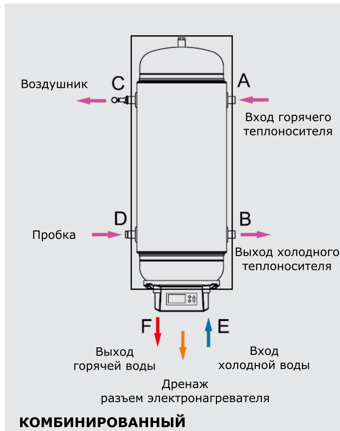
Схема устройства бойлеров.
